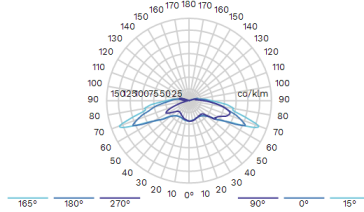
6370 asymmetrisch (schmalstrahlend)
